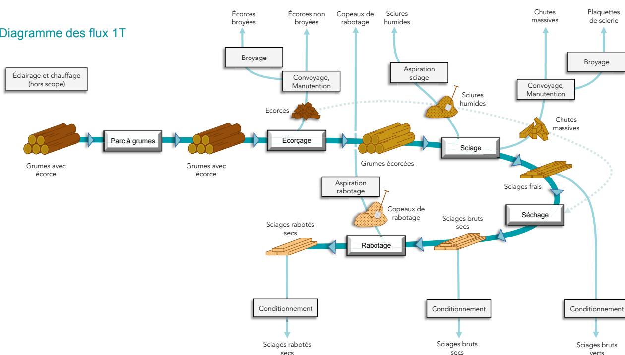
Schéma synthétique des processus et flux de produits de première transformation
